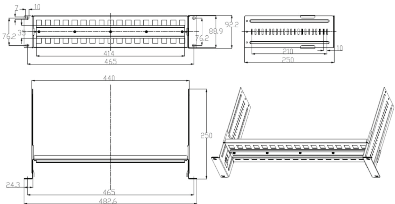
2U DIN Rail mounting frame
